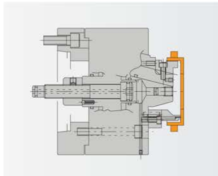
● YOKE FLANGE
