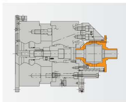
● CASE
